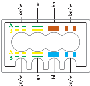
Конфигурация по TIA/EIA 568 B
