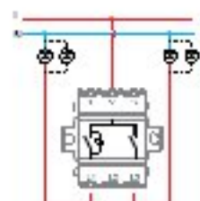
клуч сх. 5 светил switch 2 gang 1 way - light 250V, 10A, IP20
