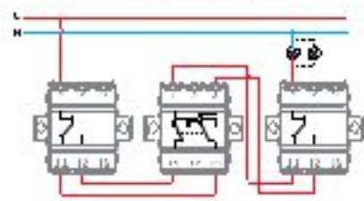
клуч крестов сх. 7 switch intermediate 7 250V, 10A, IP20
