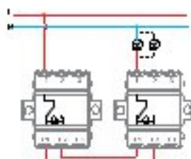
клуч сх. 6 светил switch 1 gang 2 way - light 250V, 10A, IP20
